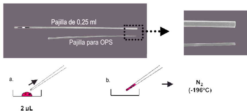
Figura 2. Pajilla abierta y estirada ( Open pulled straw , OPS), pajilla de 0,25ml. a. Gota de 2 \mu l de crioprotector con los oocitos. b. Montaje de la gota por capilaridad en la pajilla y su paso directo al nitrógeno líquido. Fuente: adaptado de Guignot (2005).
